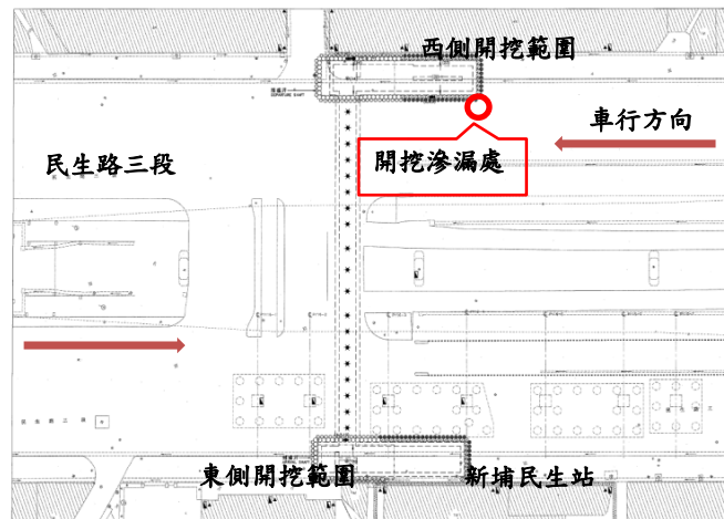
圖1 新埔民生站地下道工程開挖滲漏處
