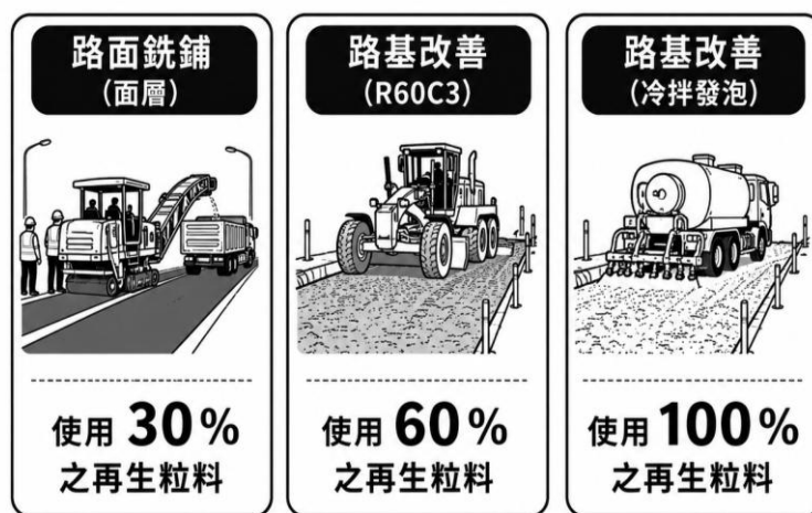
圖1 再生瀝青混凝土道路施工工法
