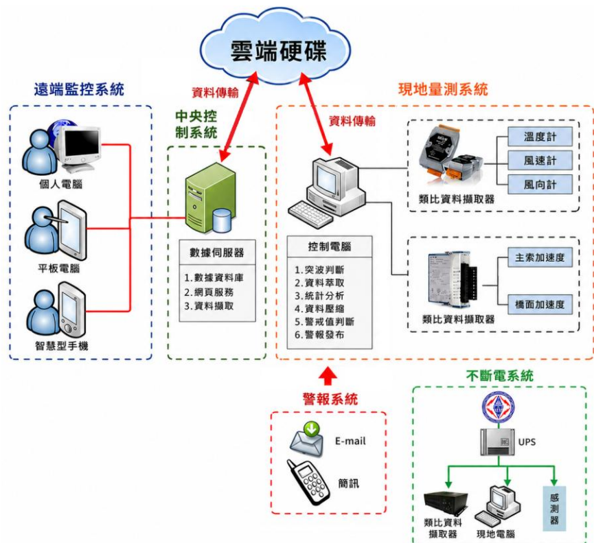
圖 3 吊橋監測系統架構
