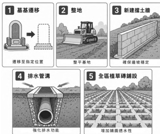
圖 3 公墓遷葬改建停車場施工情形
