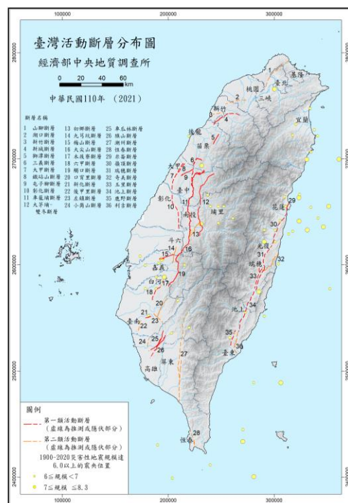
圖 1 臺灣活動斷層分布示意
