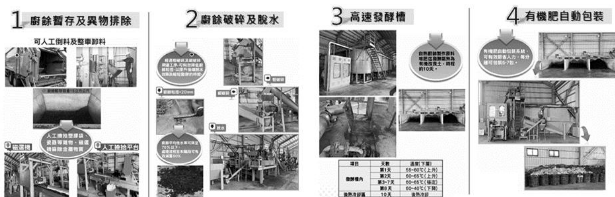
圖 3 廚餘高速發酵廠處理流程
