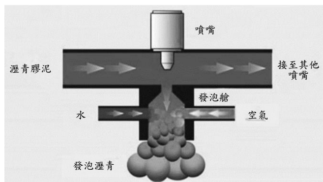
圖 1 冷拌再生瀝青發泡穩定工法
