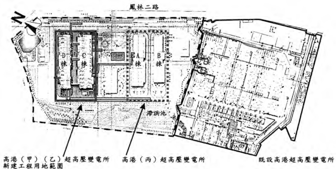
圖 5 既設高港超高壓變電所及遷改建與擴建工程用地示意圖
